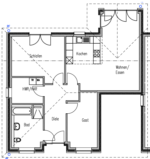
Beispielgrundriss 3-Zimmer
