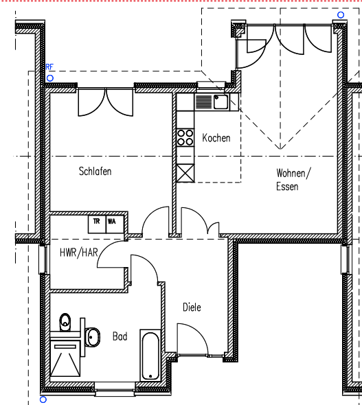
Beispielgrundriss 2-Zimmer
